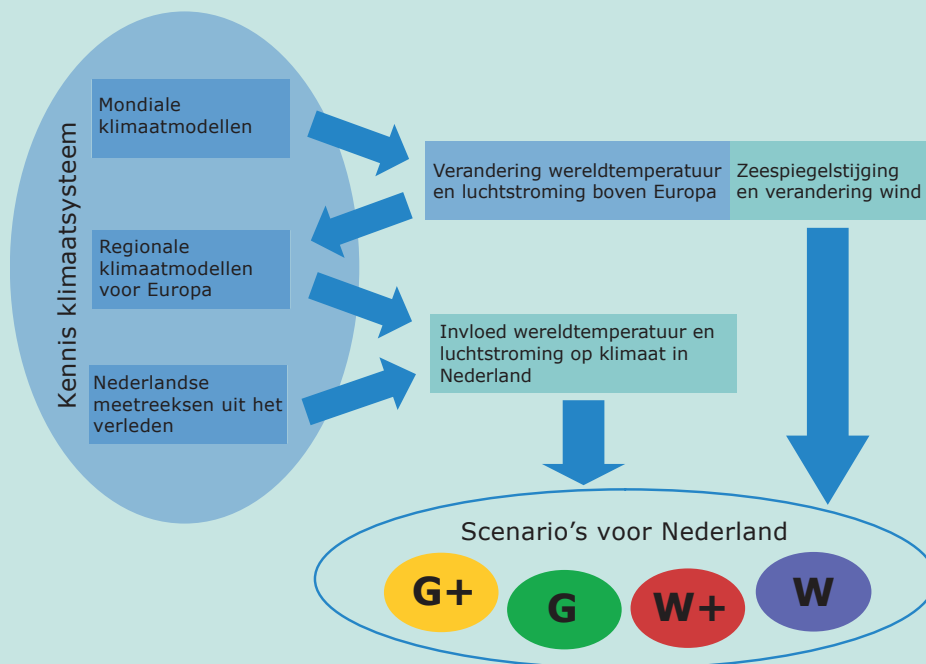
► Figuur 20 Schematische weergave van de gebruikte methode voor het afleiden van de KNMI'06 klimaatscenario's. De blauwe vakken beschrijven het bronmateriaal voor de scenario-informatie in de groene vakken. De pijlen symboliseren de informatiestroom. Voor de scenario's is gebruik gemaakt van kennis van het klimaatsysteem op mondiale, regionale en lokale schaal.
